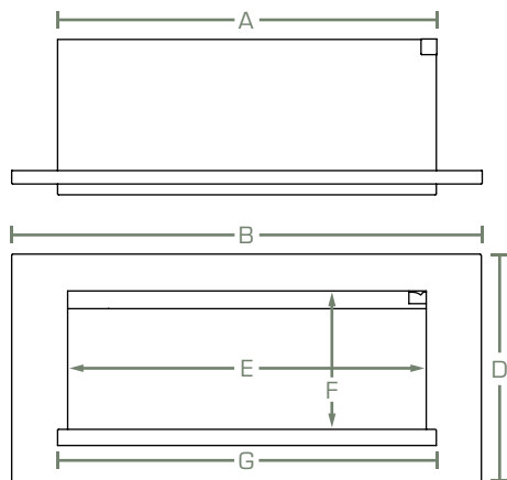
Holbury 870
